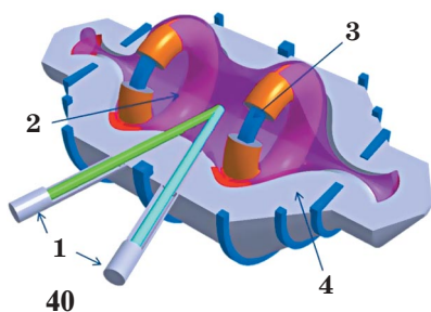
Схема компактного реактора фирмы Lockheed Martin.
